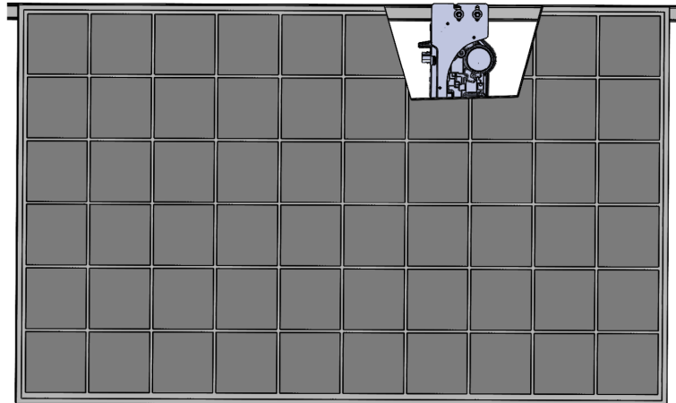
Illustration 3 : Montage horizontal
