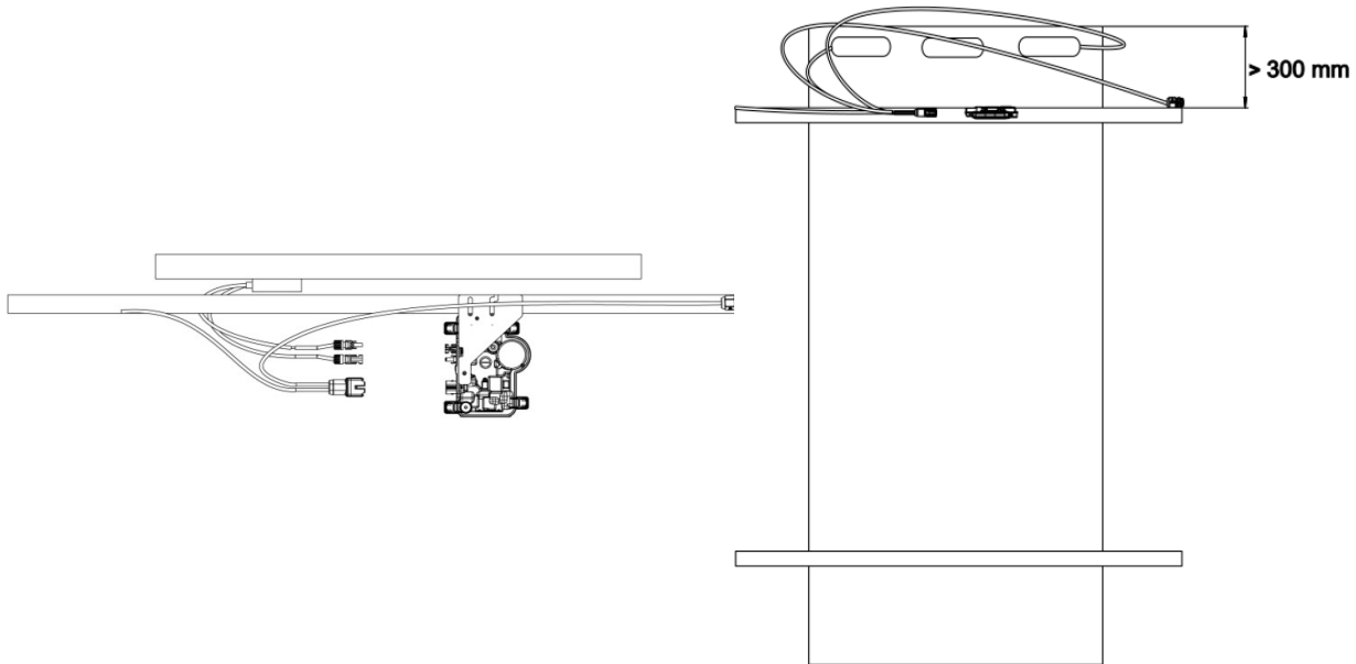
Illustration 2 : Montage vertical
