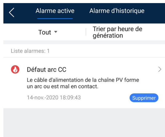
Figure 7-14 Gestion des alarmes
